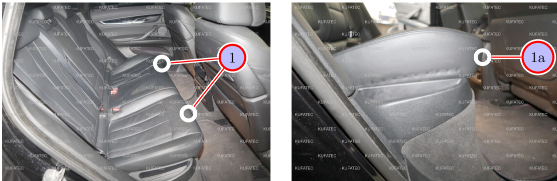
Abbildung 5: Demontage Rücksitzbank
