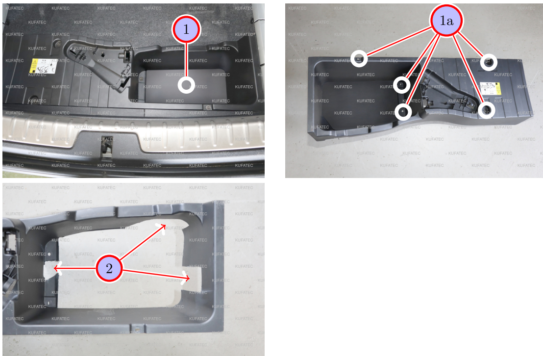
Abbildung 8: Anpassung Kunststoffablage Kofferraum
