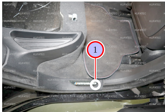
Abbildung 6: Demontage Einstiegsleiste Beifahrerseite hinten
