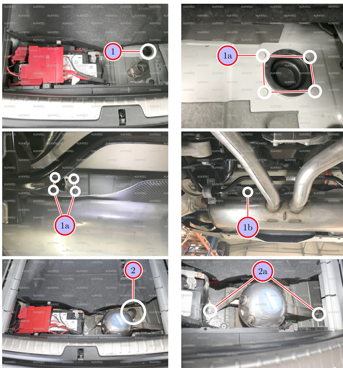
Abbildung 9: Montage Geräuscherzeuger
