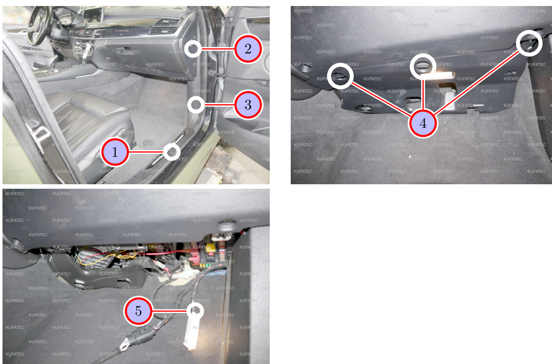
Abbildung 4: Demontage Verkleidung Beifahrerseite vorne
