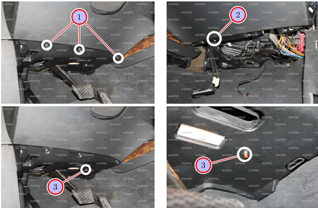
Abbildung 12: Montage Taster
