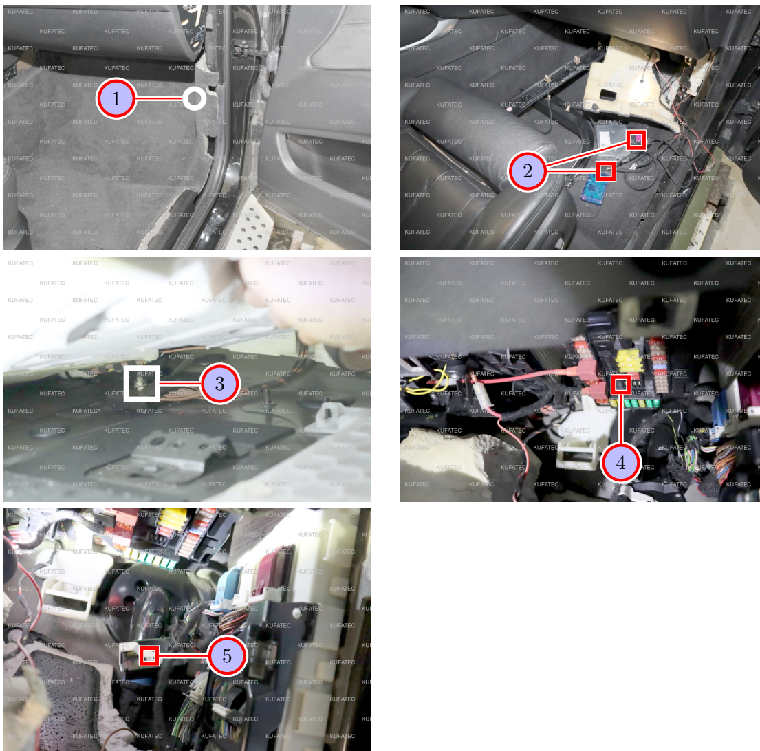
Abbildung 10: Anschluss im Beifahrerfußraum
