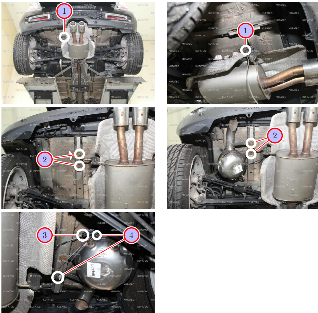
Abbildung 8: Montage / Anschluss Geräuscherzeuger
