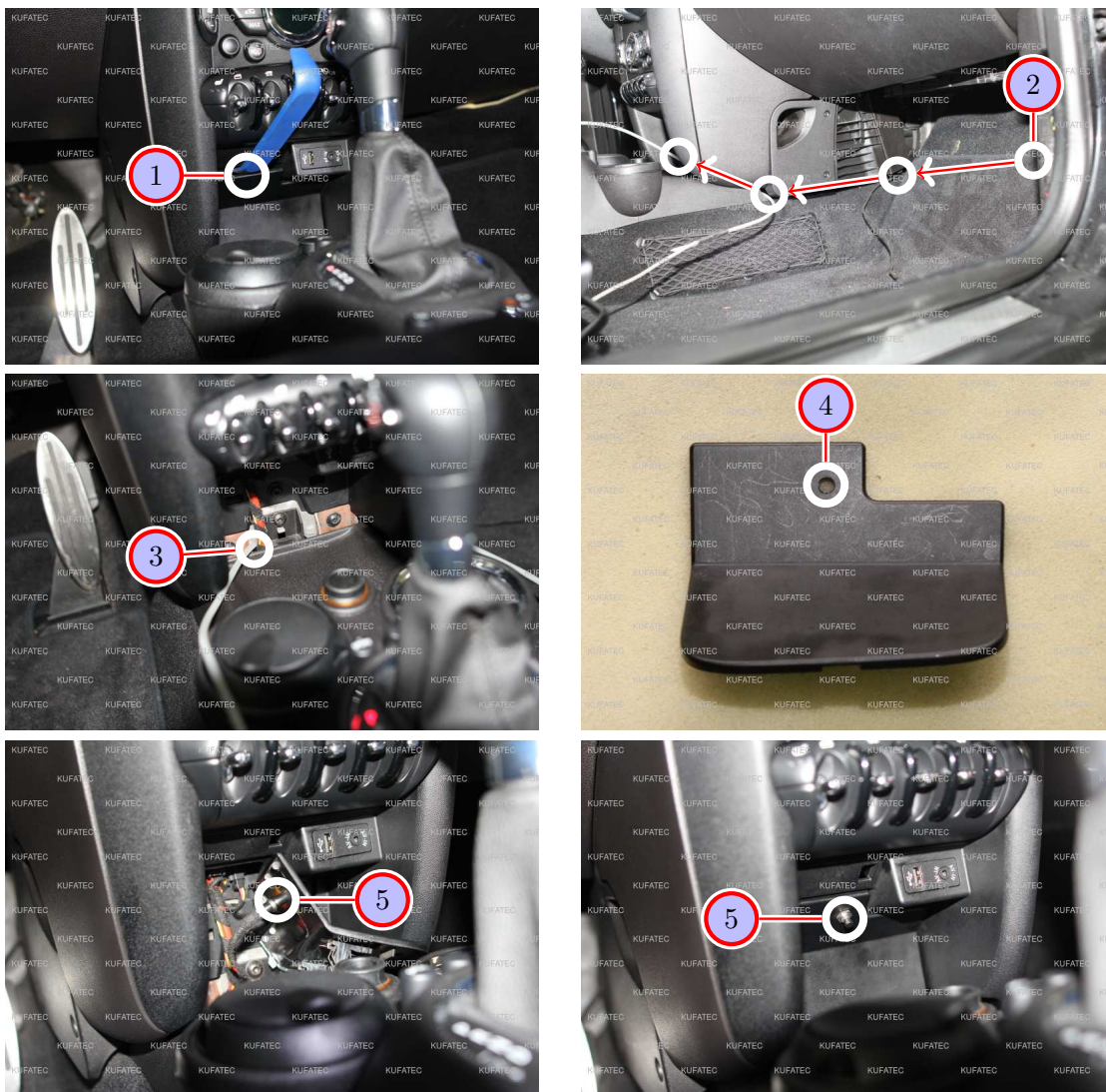
Abbildung 9: Montage Taster
