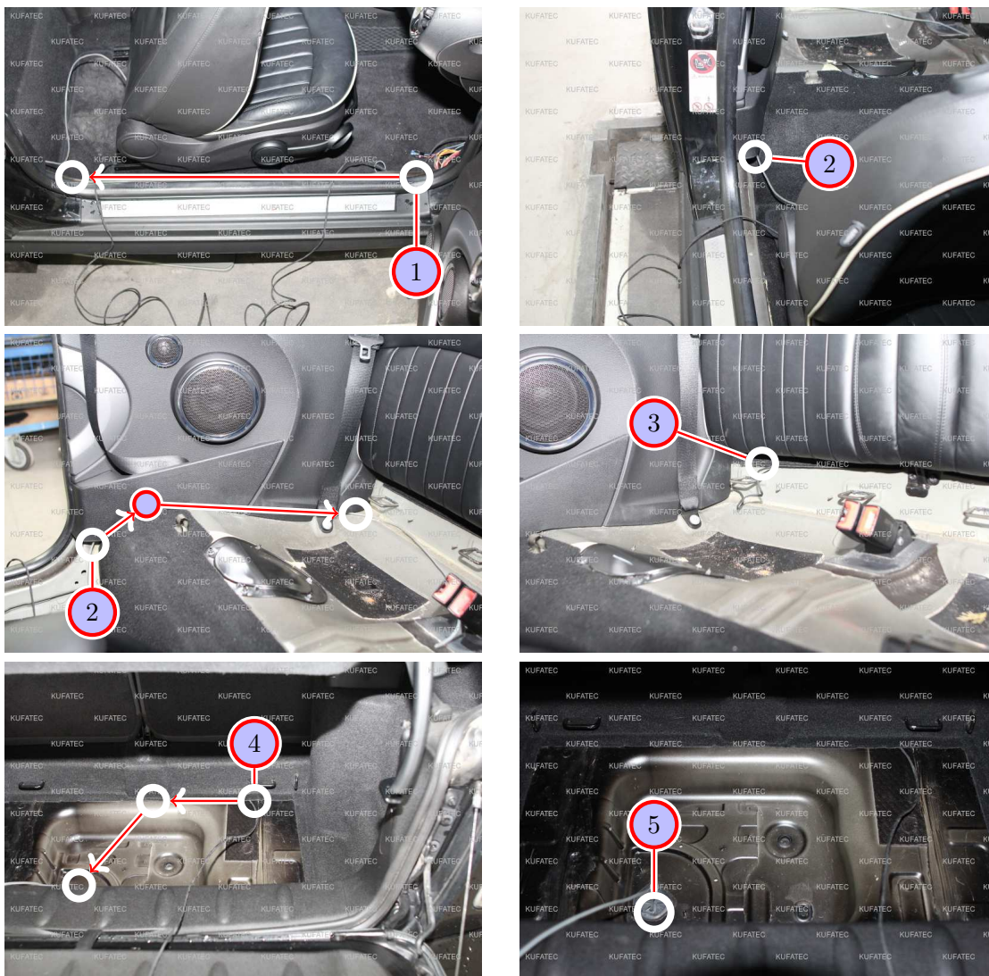
Abbildung 7: Leitungsverlegung zum Geräuscherzeuger
