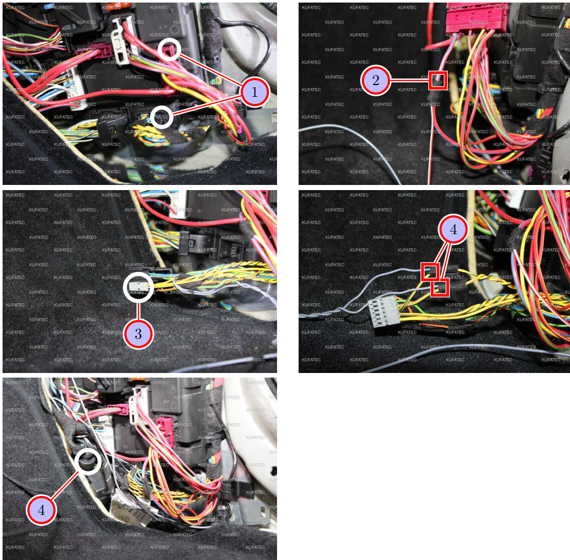
Abbildung 5: Anschluss Kabelsatz
